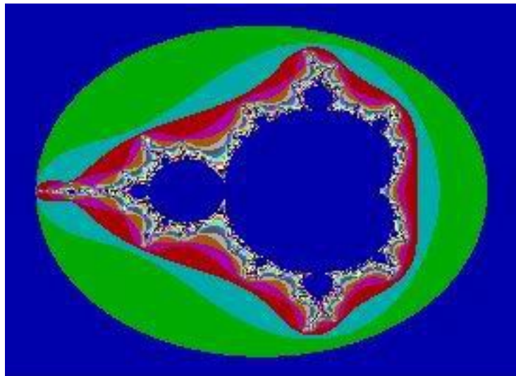
Серия Манделброта
